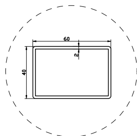
PROFILO ORIZZONTALE
