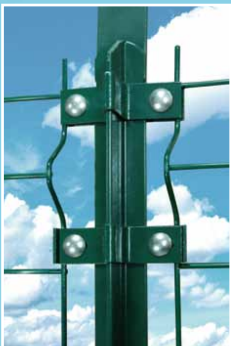
fissaggio pannelli
