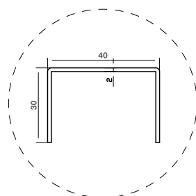
PROFILO ORIZZONTALE
