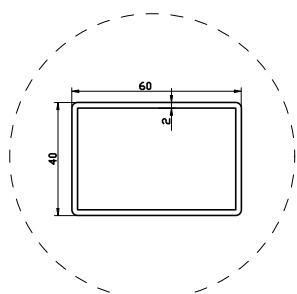
PROFILO ORIZZONTALE
