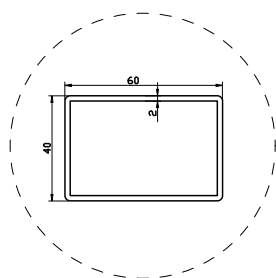
PROFILO ORIZZONTALE
