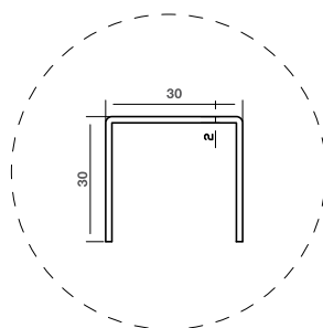
PROFILO ORIZZONTALE
